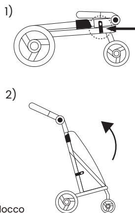
Shema 6. Blocco di sicurezza
